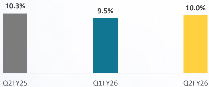
EBITDA Margins (%)
