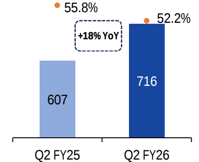
RoCE (%), TTM 2
